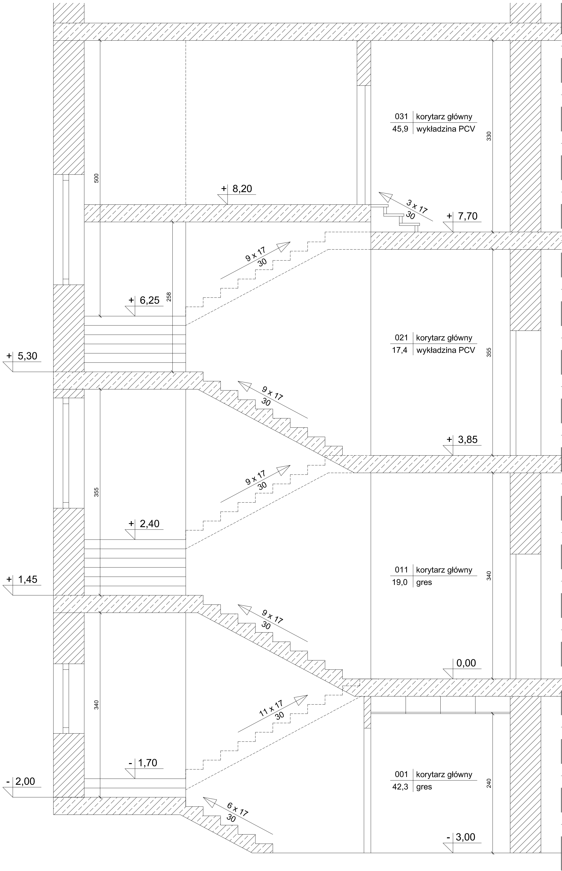
Pzekrój A-A
